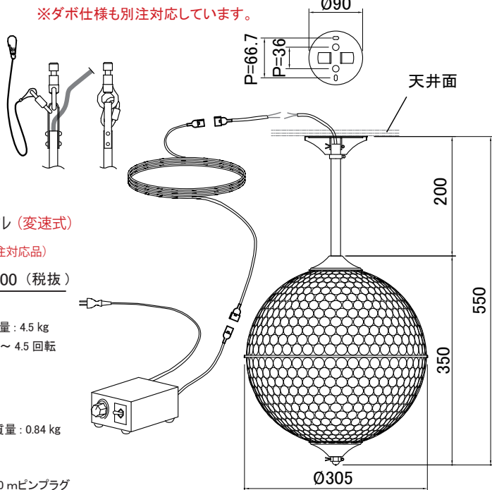
■据置吊下兼用丸鏡ミラーボール (変速式) NMB-3599P (受注対応品) ¥176,000 (税抜)
