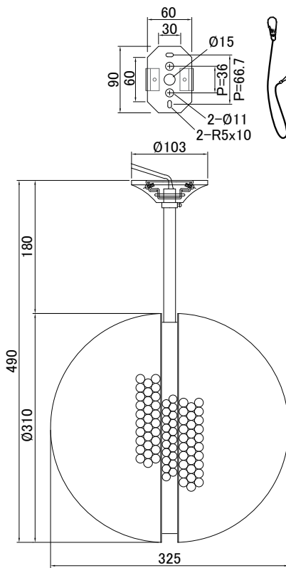
NMB-3543P ダボ仕様取付部図
