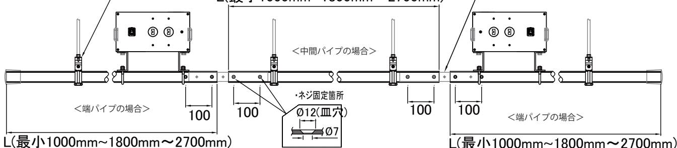
吊金具
