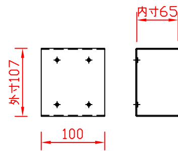
連結金具 1ヶ
