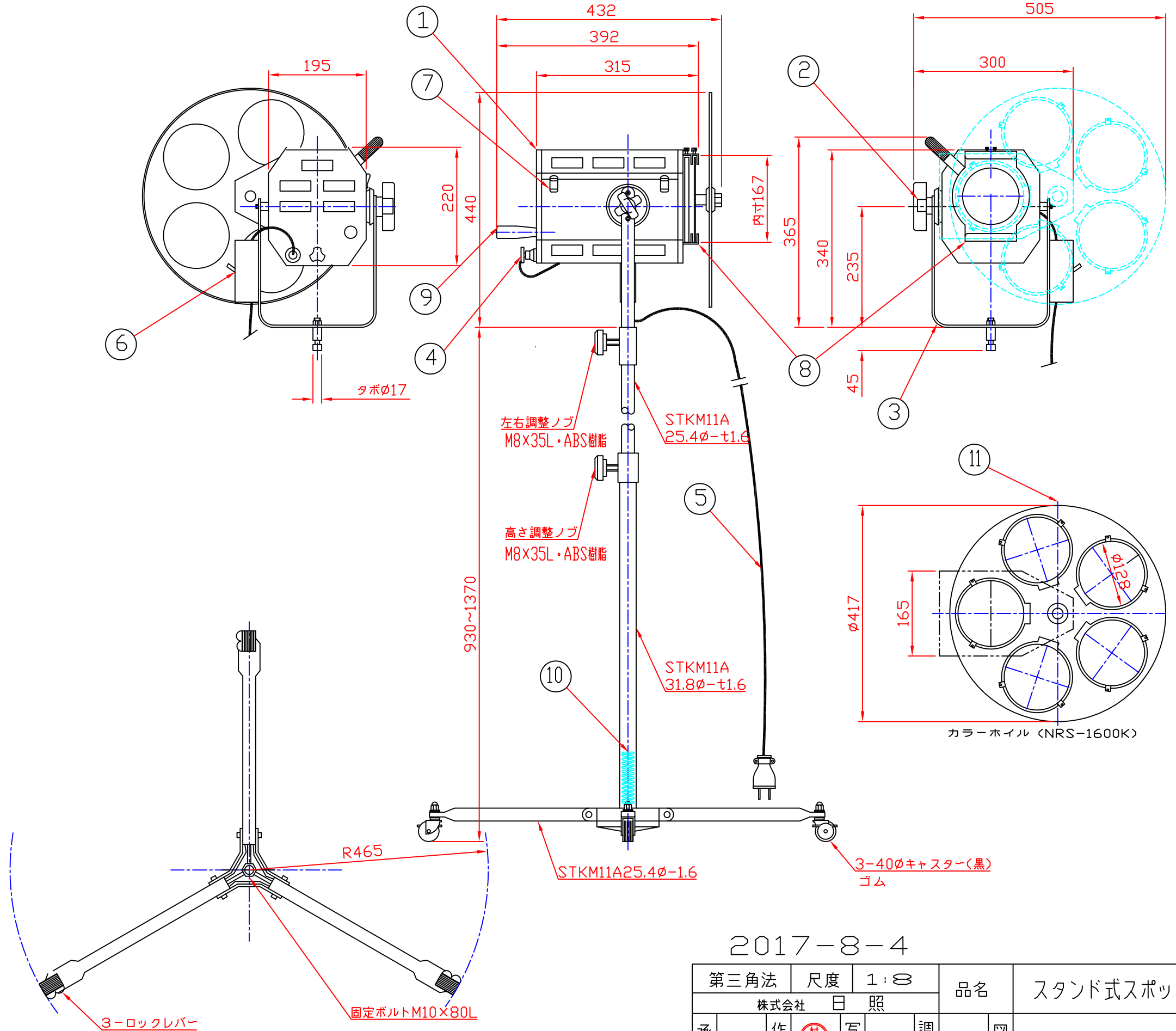
三脚スタンド (NRS-1548K)
