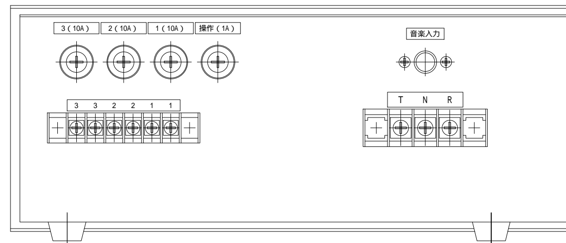
裏面詳細
