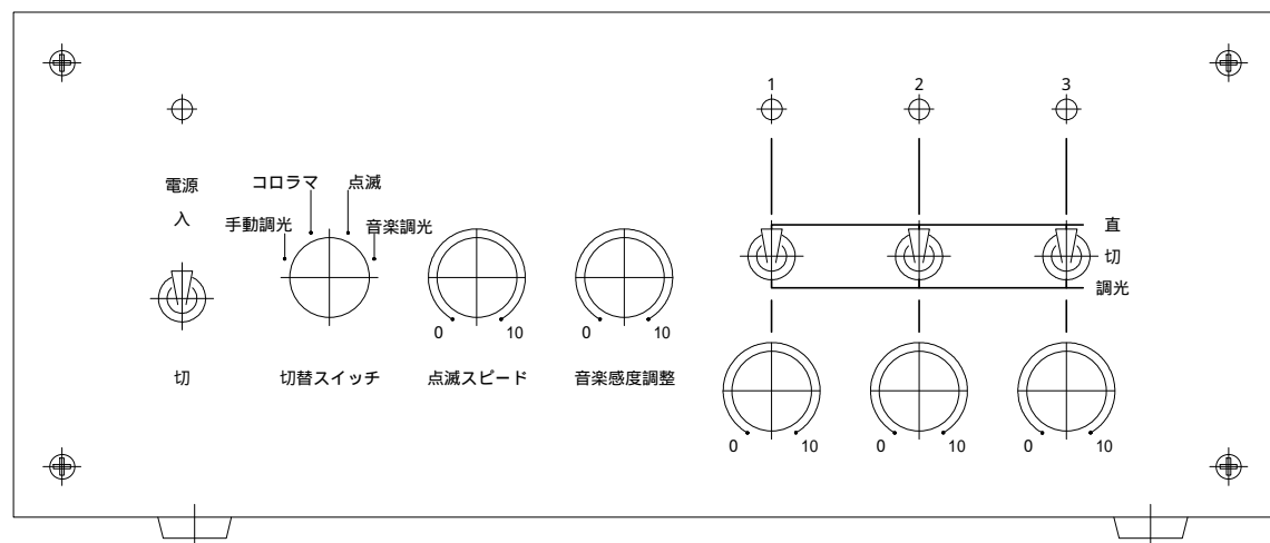
正面詳細
